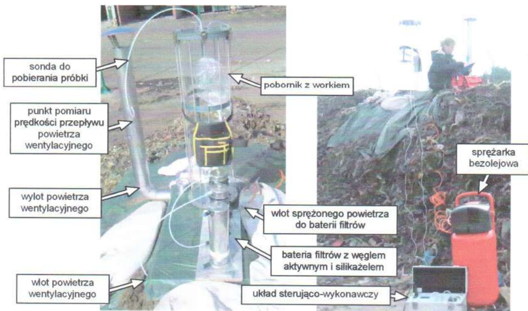
Rysunek 10. Pobieranie próbek powietrza z nad powierzchni przyzmy
