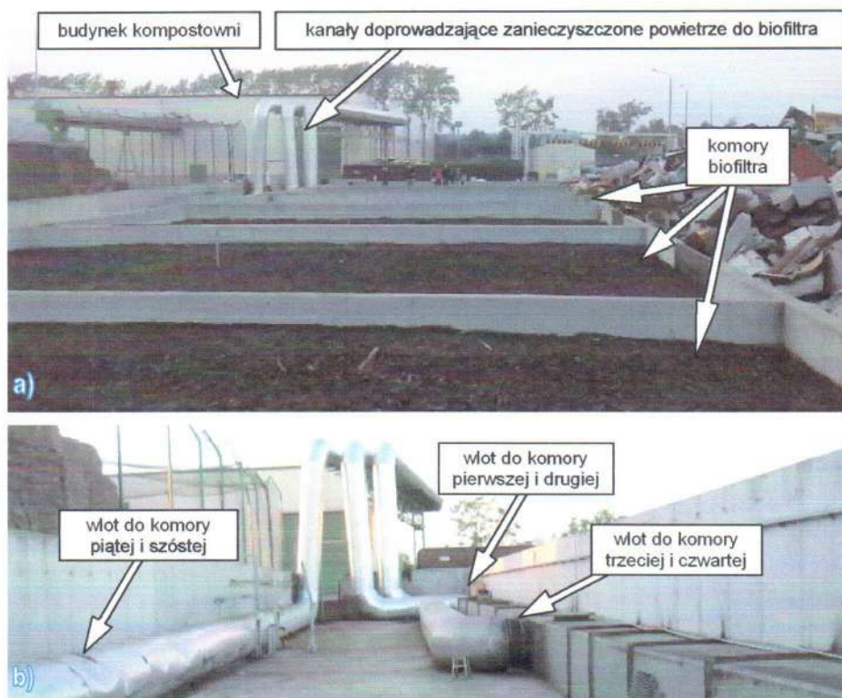
Rysunek 1. Biofiltr
